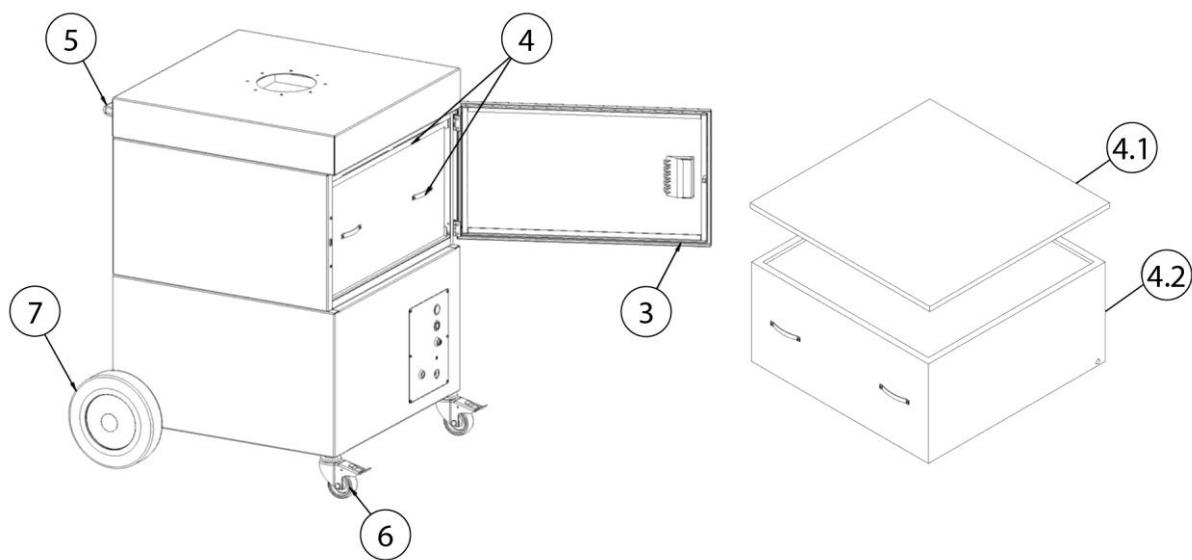
Sl. 4: Montaža
